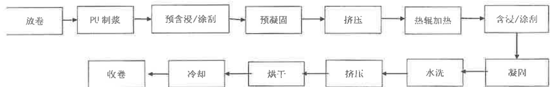
图 33-5 聚氨酯湿法生产工艺流程图
