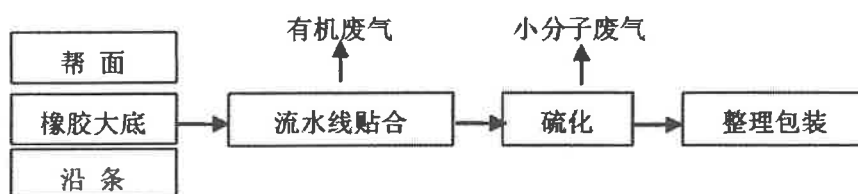
图 35-6 硫化工艺-帮底装配单元工艺流程图
