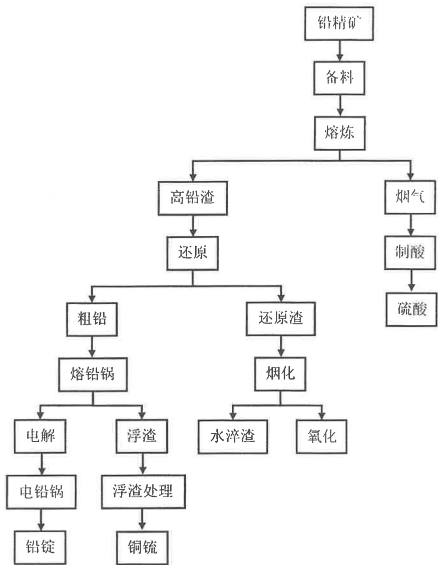
图 11-1 铅冶炼典型生产工艺流程图
