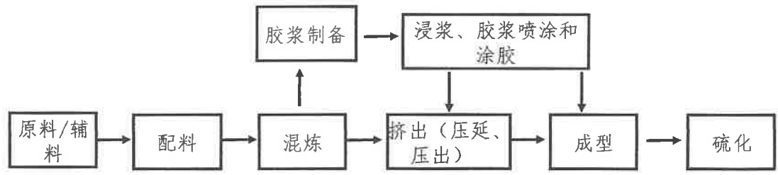
图 34-2 橡胶板、管、带制品制造工艺流程图
