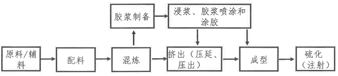
图 34-3 橡胶零件、运动场地用塑胶及其他橡胶制品制造工艺流程图
