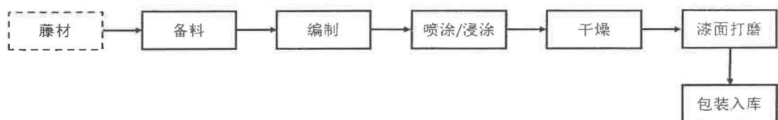
图 36-3 典型藤家具制造生产工艺流程图
