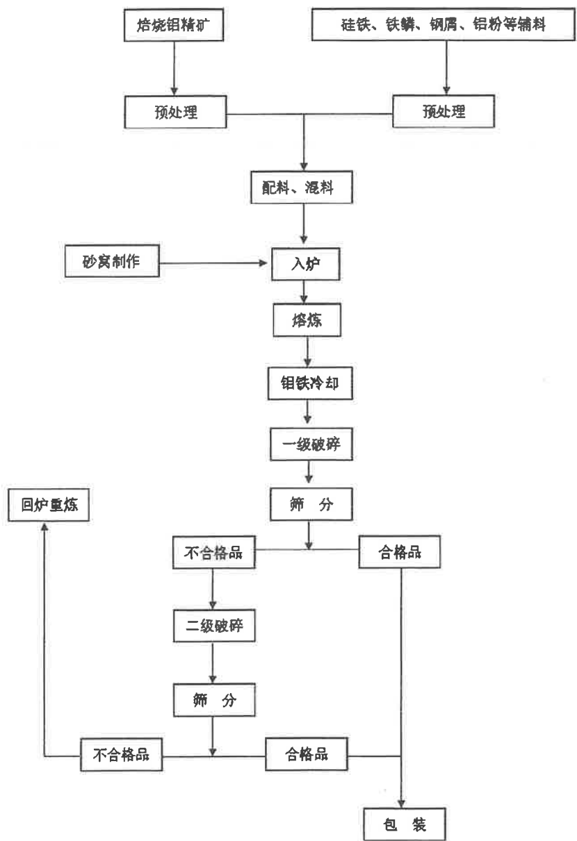
图 12-2 钼铁典型生产工艺流程图
