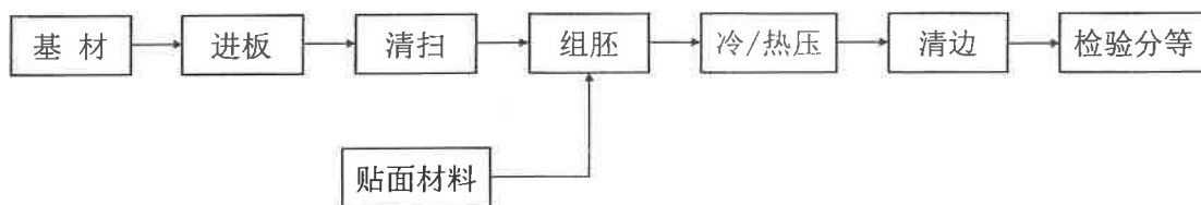
图 32-5 饰面人造板制造生产工艺流程图
