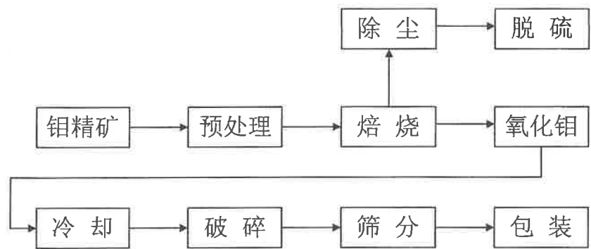
图 12-1 焙烧钼精矿典型生产工艺流程图
