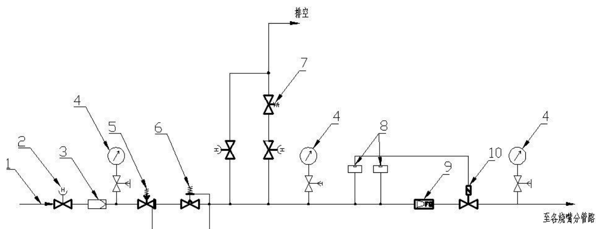
图 C.1 燃烧系统主管路构成示意图
