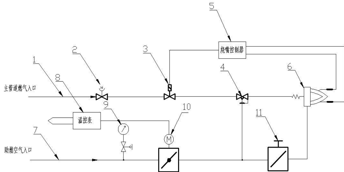
图 D. 1 燃烧系统支管路构成示意图
